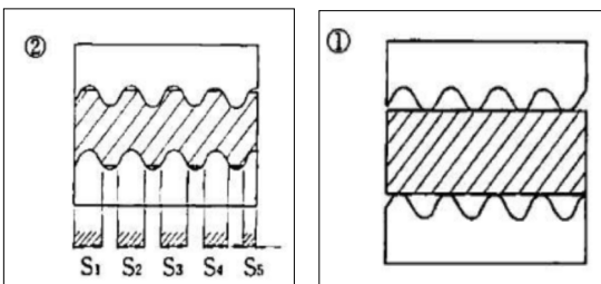
面圧良好 なじみが良く密封可
